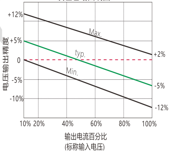
5VDC/12VDC/24VDC输入/3.3VDC输出 误差包络曲线图
