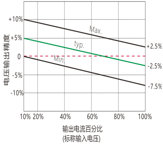
3.3VDC/5VDC输入/其他输出 误差包络曲线图
