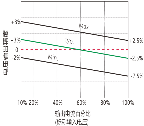
12VDC/15VDC/24VDC输入/其他输出 误差包络曲线图
