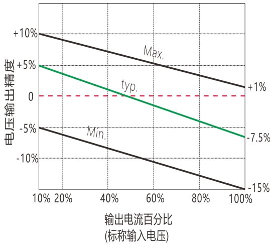
3.3VDC输入/3.3VDC输出 误差包络曲线图
