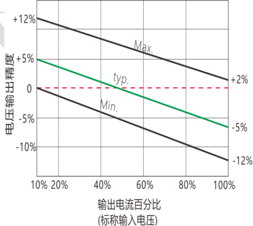
5VDC/12VDC/24VDC输入/3.3VDC输出 误差包络曲线图
