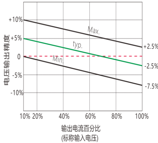
3.3VDC/5VDC输入/其他输出 误差包络曲线图
